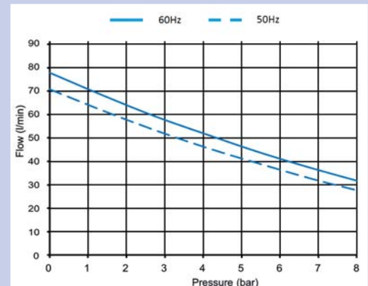
Modell 87R-25B
